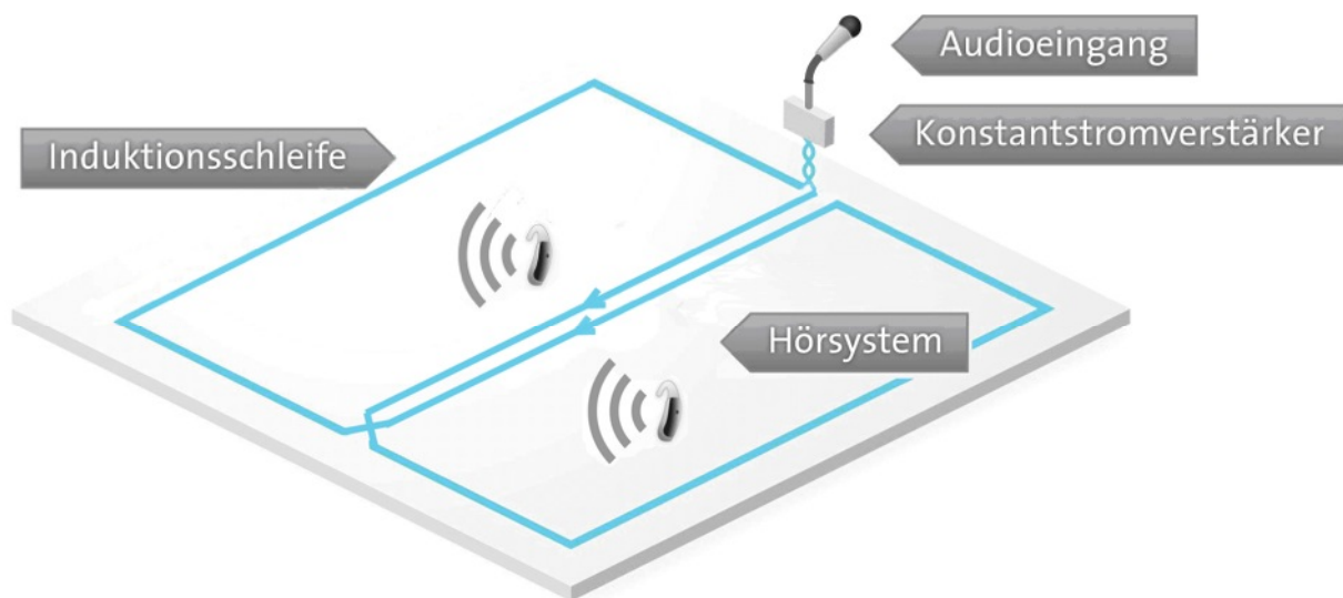
Abbildung 5 : Schematischer Aufbau eines Mehrsegmenteschleifensystems
