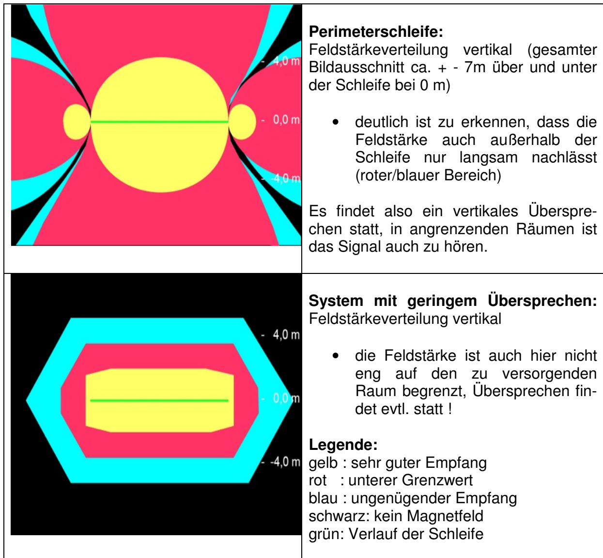
Abbildung 3 : Vergleich der vertikalen Feldstärkeausbreitung zwischen einer Perimeterschleife und einem Mehrsegmenteschleifensystem mit Phasenschieber und geringem Übersprechen.
